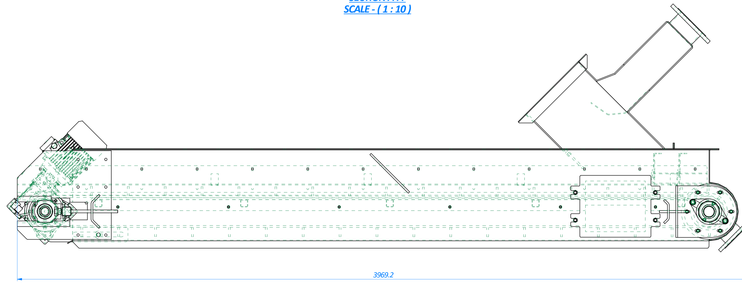
SCALE - (1 : 10)
