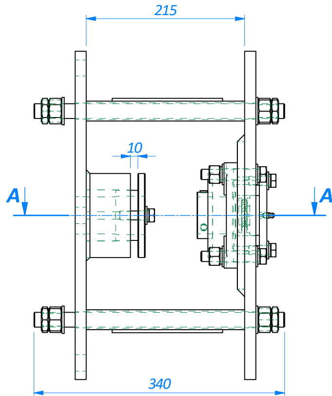
SCALE - (1 : 5)
